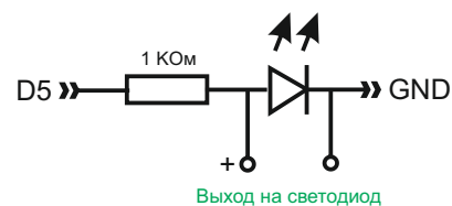
Сигнальный светодиод
