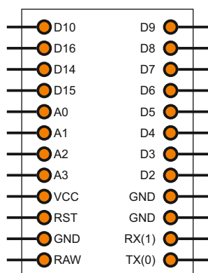
Arduino Pro Micro
