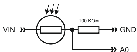
Фоторезистор
