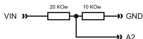
Контроль напряжения
