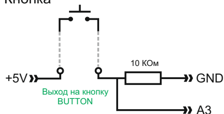
Кнопка
