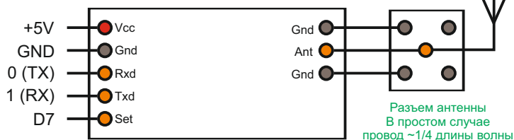
Разъем для подключения радиомодуля HC-12 / SV610
