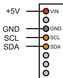
Разъем для подключения платы датчиков GY-91
